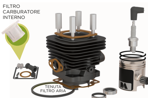
KIT PISTONE CILINDRO E MANUNTENZIONE
